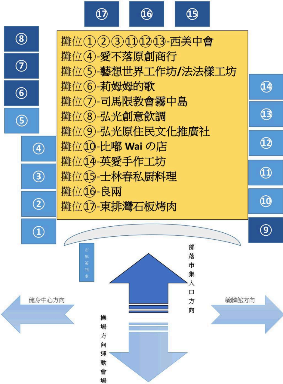
Patiyaman 部落市集現場平面圖
